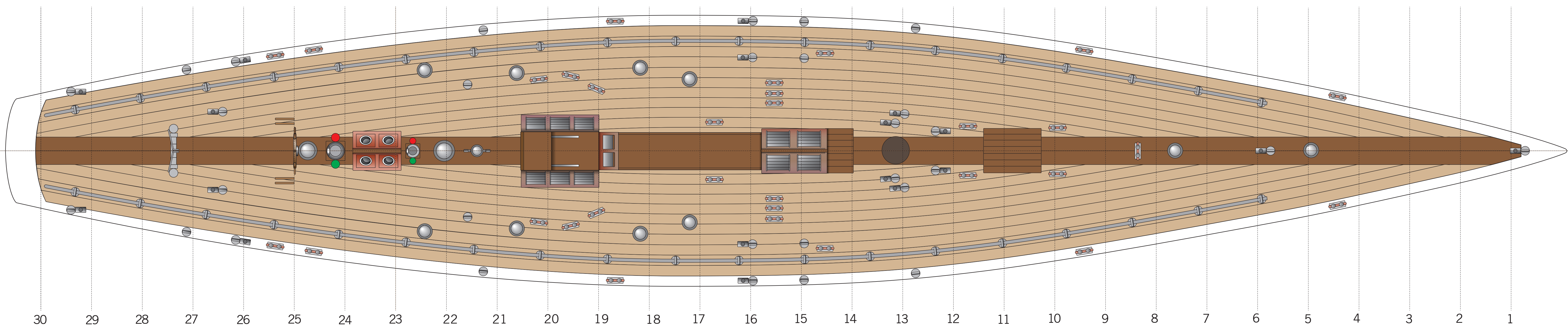
RAINBOW J5 VAINQUEUR DE L'AMERICA CUP EN 1934 Échelle 1/45 Plan dessiné par Serge Ducruit Planche 1/2
